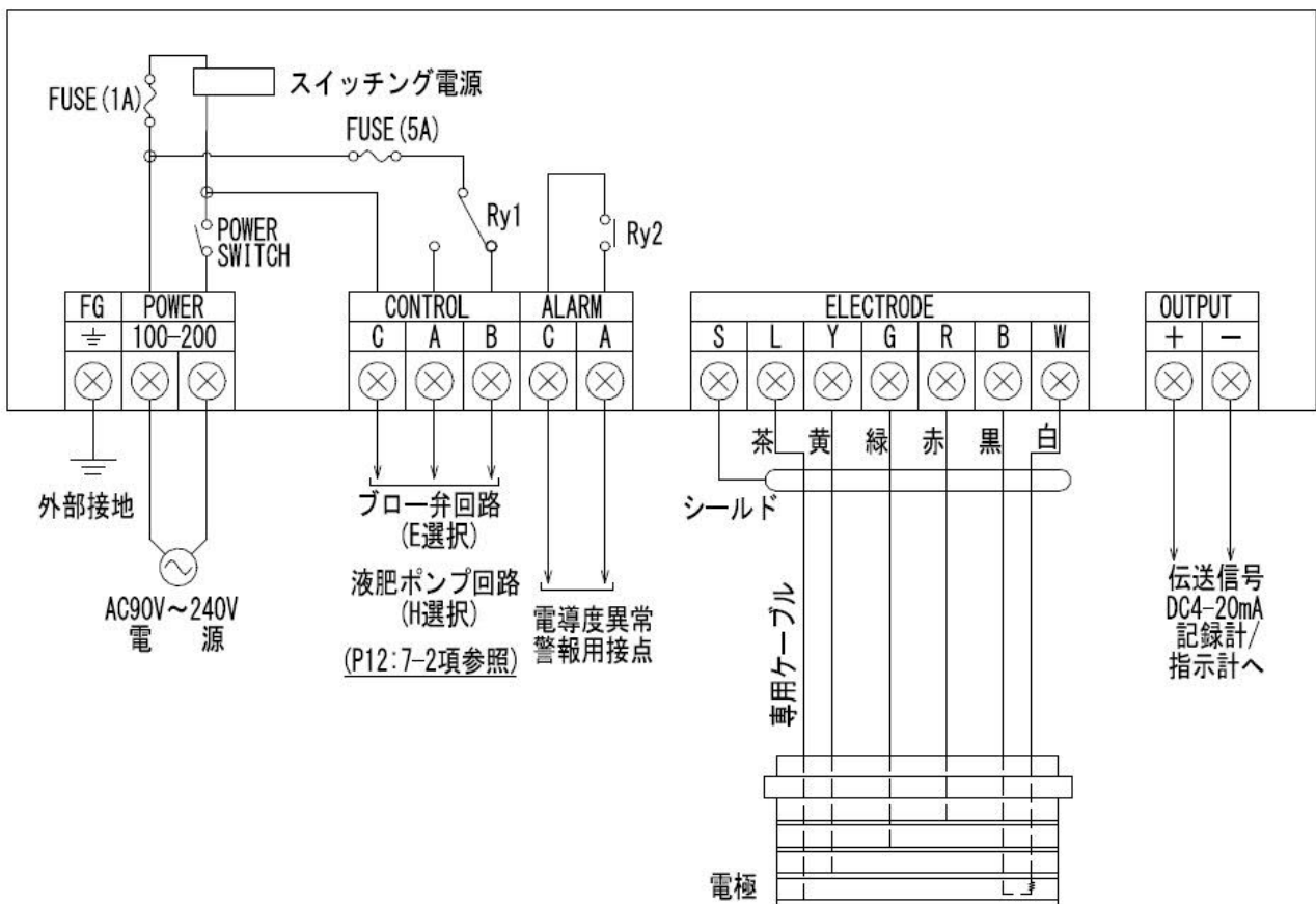
外部端子接続図
