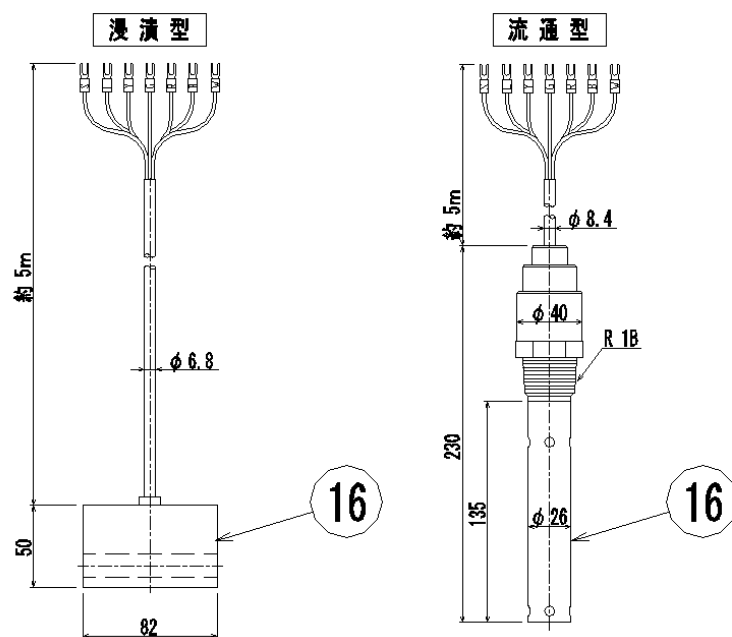
⑯ 電極センサー（本体） 4電極式
