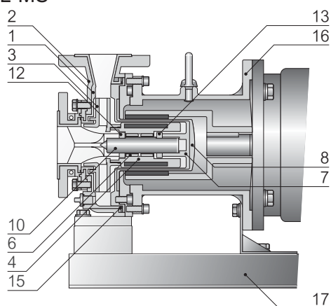
TSL-MS
