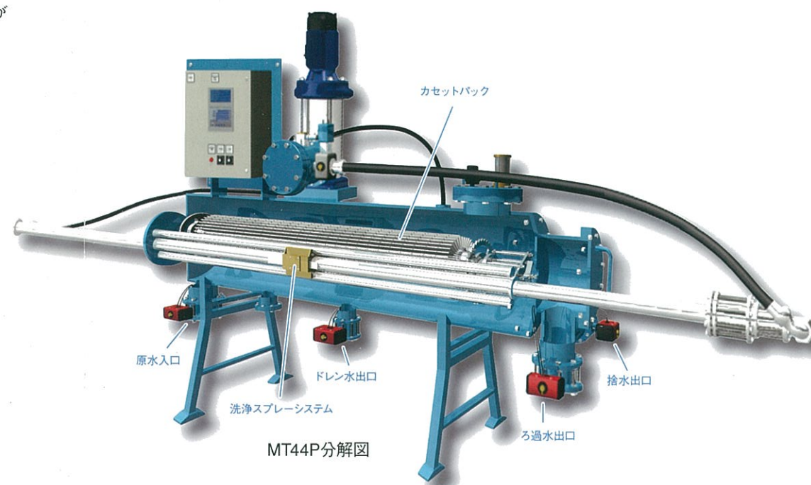
図1: 洗浄スプレーシステムとカセットパック
