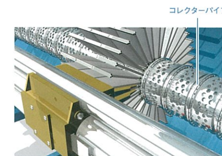
図1: 洗浄スプレーシステムとカセットパック
