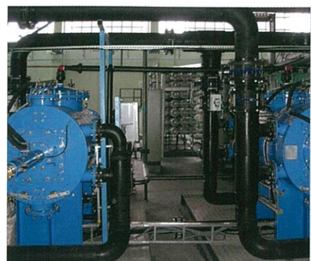
MTG×2台並列設置 (RO膜前処理・日量5,500m³処理)
